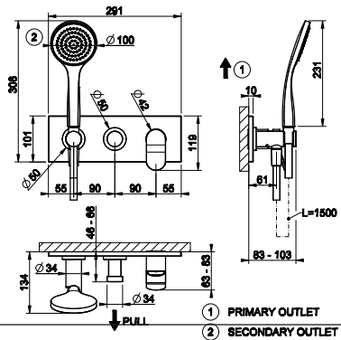
56041 External part wall-mounted two ways shower mixer with handshower. Parte esterna miscelatore doccia a parete 2 vie con doccetta.
